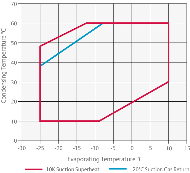
ZS*KA - R448A/R449A
