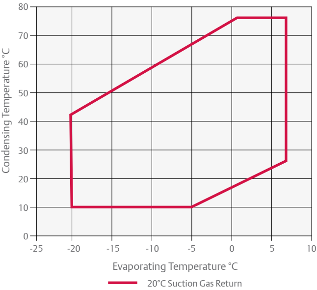
ZS*KA - R134a
